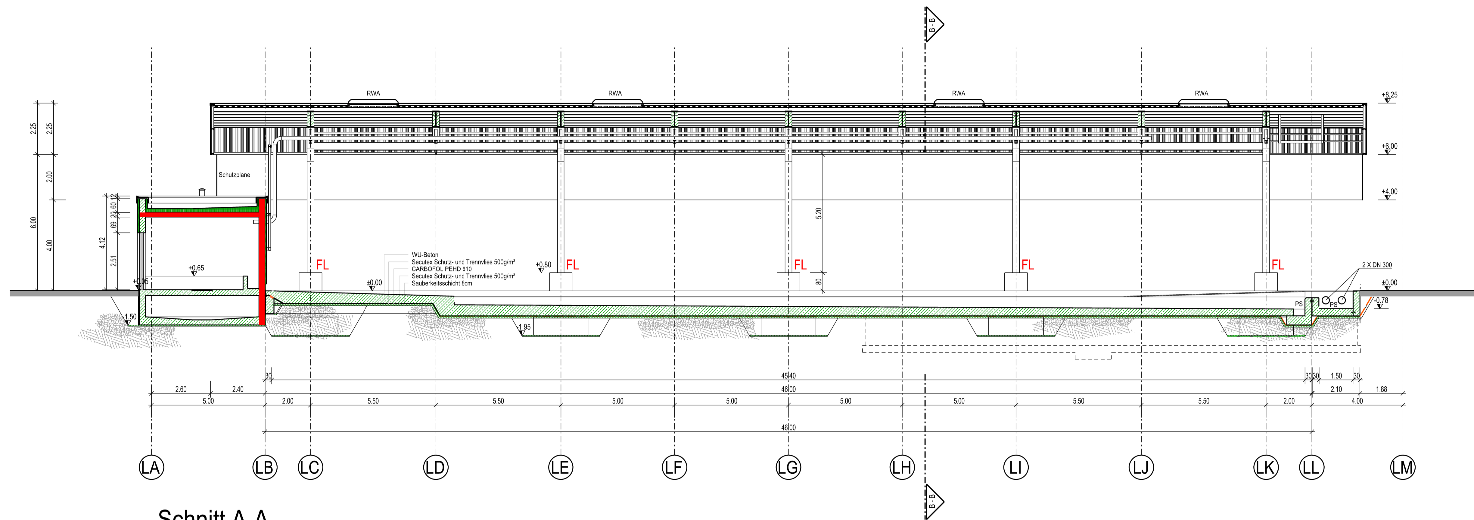
Schnitt A-A
