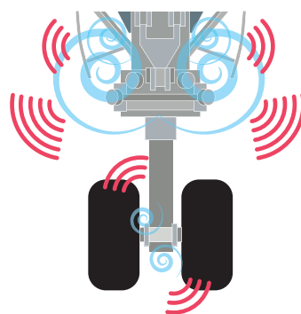
Ohne Fahrwerkverkleidung
