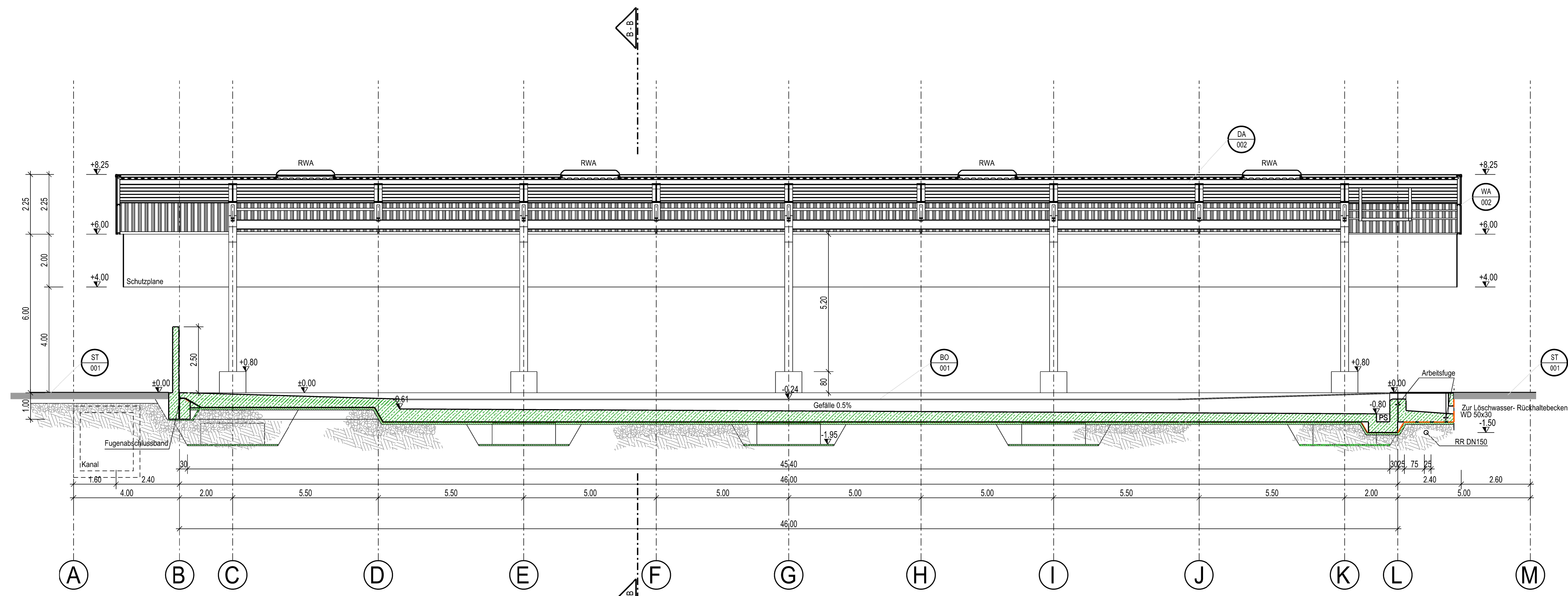
Schnitt A-A
